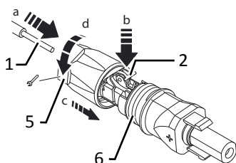
Rys. 18: Wprowadzić żyły
