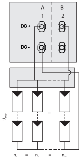
Imm. 23: Un generatore in parallelo su entrambi gli inseguitori MPP
