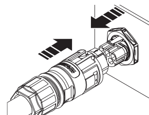
Afb. 17: AC-aansluitstekker met de stekker van het apparaat verbinden
