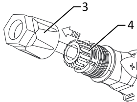
III. 19: Pousser l'insert dans le manchon
