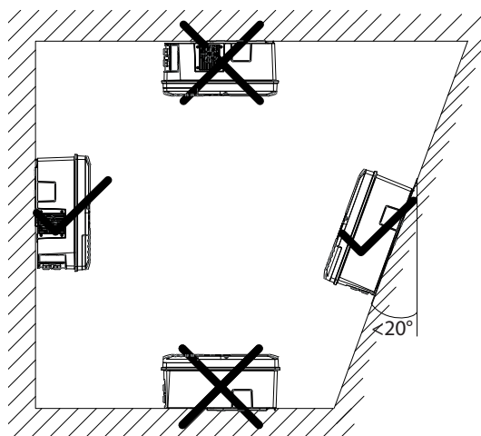
Fig. 4: Posição de instalação permitida
