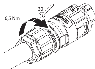
Fig. 15: Apertar o buçim roscado
