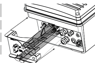
Fig. 26: Fechar a tampa de ligação
