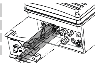
Fig. 26: Cierre la tapa de conexión
