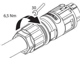
Afb. 15: Kabelwartel vastdraaien
