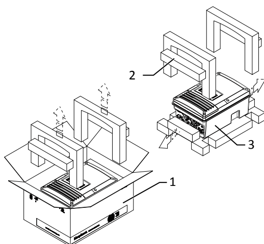
Abb. 5: Gerät auspacken
