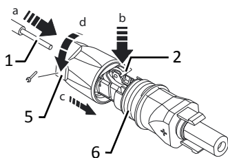
Fig. 18: Introducir los conductores
