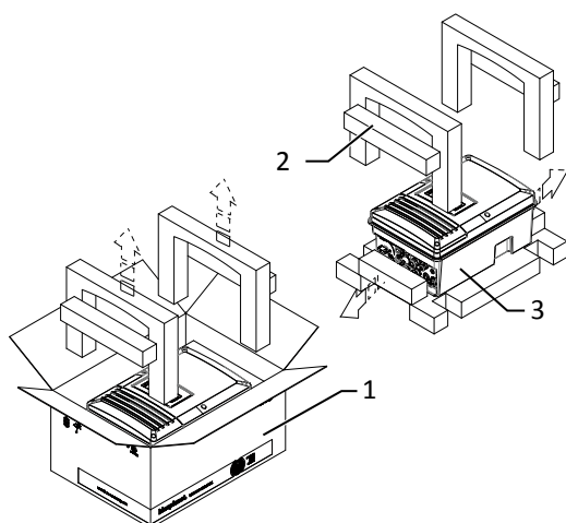
Afb. 5: Apparaat uitpakken
