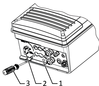
Rys. 9: Odslanianie przyłączy DC
