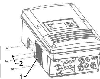
Abb. 27: Lüfter ausbauen
