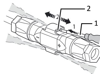
Fig. 32: Saque el conector
