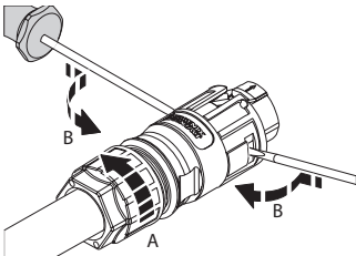
Abb. 29: Gehäuse öffnen und Leitungen lösen
