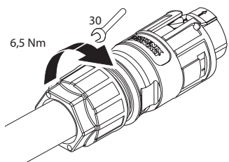
Fig. 15: Apriete el racor de cable
