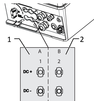
Rys. 24: Przyłącze bieguna dodatniego i ujemnego DC
