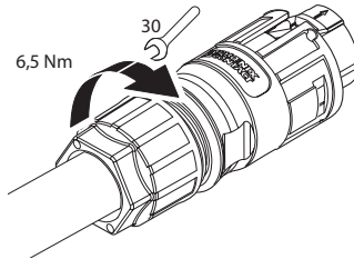
Şek. 15: Kablo rakorunun sıkılması
