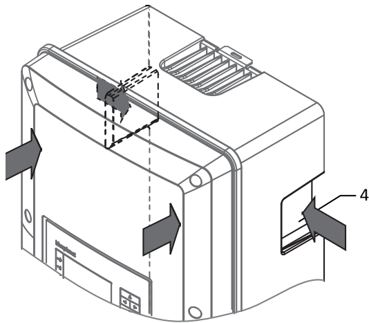
Fig. 6: Levante el equipo
