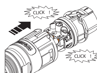
Fig. 16: Pressionar suporte de contacto na caixa
