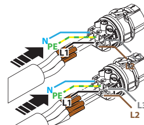
Fig. 13: Conectar os fios ao suporte do contacto
