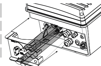
Abb. 26: Anschlussdeckel schließen
