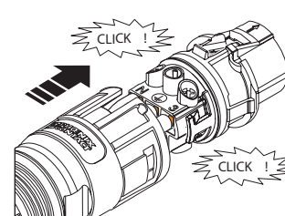
III. 16: Insérer le bornier dans le boîtier
