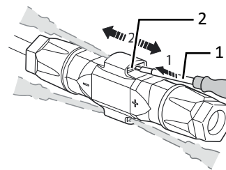
III. 32: Détacher le connecteur à fiche
