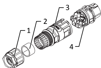
Afb. 11: AC-aansluitstekker
