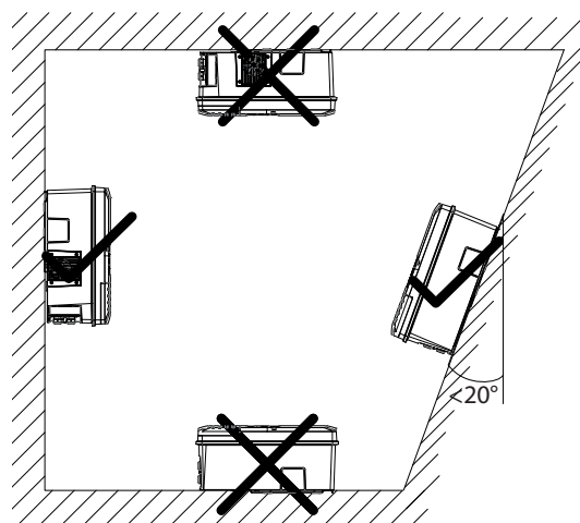
III. 4: Lieu de montage autorisé
