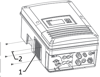
Şek. 27: Fanın sökülmesi
