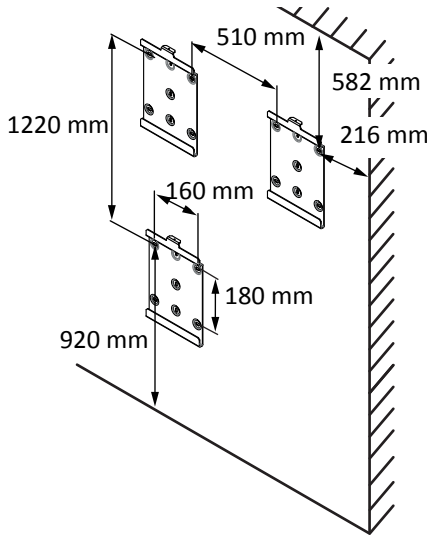
Fig. 8: Montagem na parede
