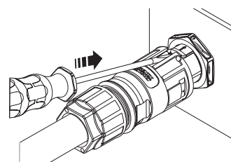
Imm. 31: Togliere il connettore CA dal connettore dell'apparecchio
