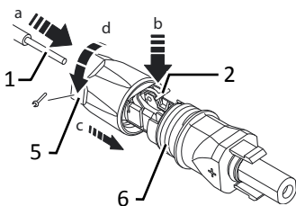
Fig. 18: Insert wires
