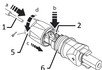
Fig. 18: Introduzir os fios
