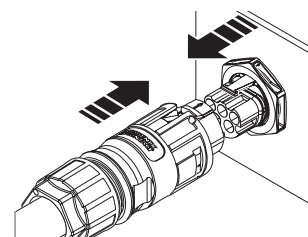
III. 17: Faire enclencher le connecteur CA avec la fiche de l'appareil
