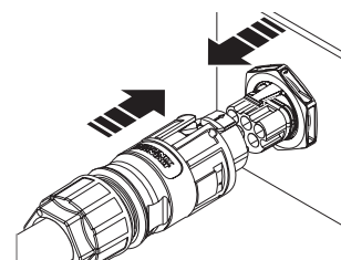
Fig. 17: Encaixar o conector de ligação CA no conector do dispositivo
