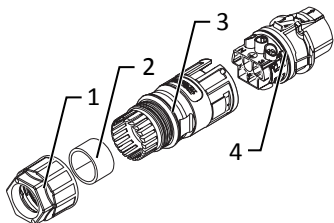
Abb. 11: AC-Anschlussstecker
