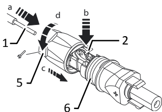
Abb. 18: Adern einfügen
