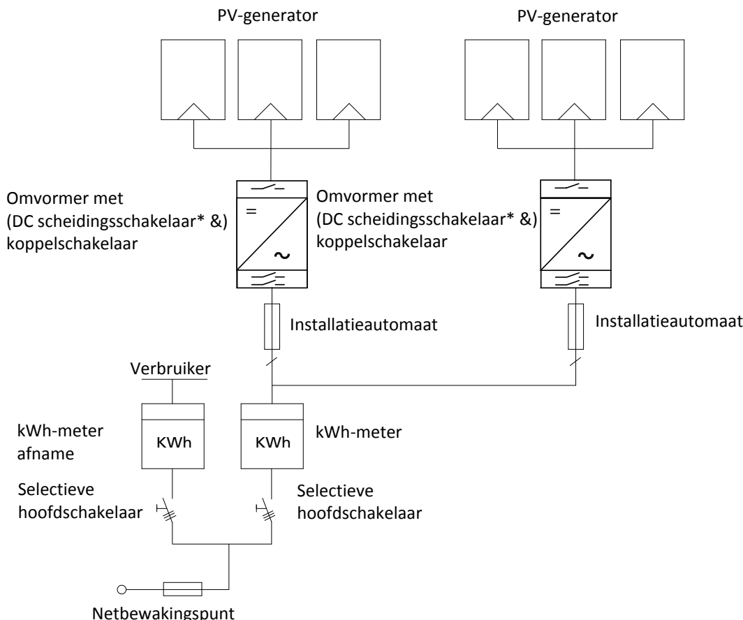
Afb. 1: Overzichtsschakelschema voor een installatie met twee omvormers
