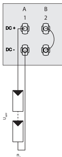
III. 22: Montage des entrées en parallèle avec adaptateur Y, court-circuitage du régulateur MPP B non utilisé
