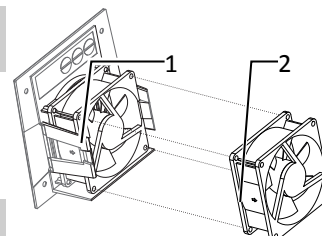
Abb. 28: Lüfter abstecken
