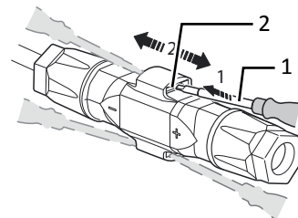
Fig. 32: Desligar os conectores
