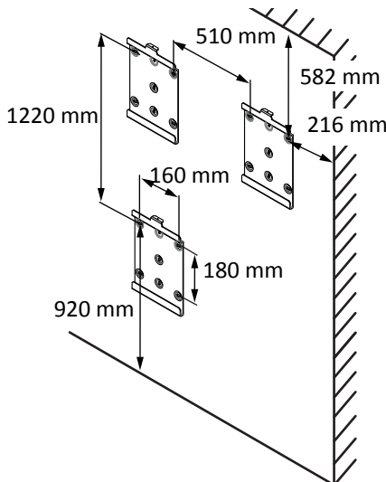
Fig. 8: Montaje mural
