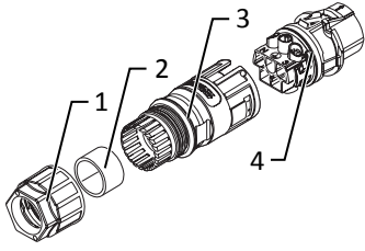
Şek. 11: AC bağlantı soketi
