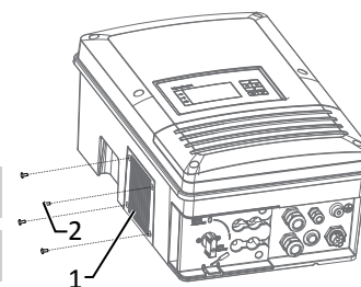
III. 27: Démontant le ventilateur
