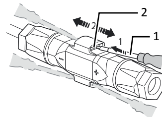
Imm. 32: Estrazione del connettore
