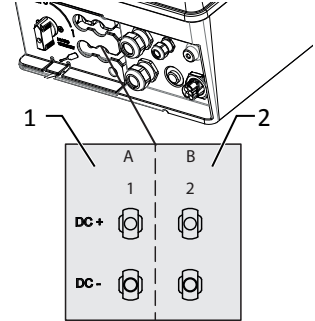
Şek. 24: DC artı ve DC eksi bağlantısı
