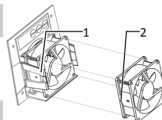
Fig. 28: Extracción del ventilador
