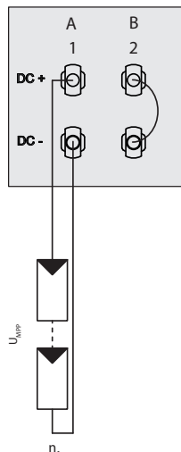
Abb. 22: Parallele Eingangsbeschtung mit Y-Adapter, Kurzschluss des nicht verwendeten MPP-Trackers B
