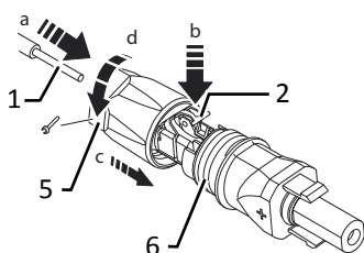
III. 18: Insérer les fils
