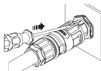
Fig. 31: Soltar o conector de ligação CA do conector de encaixe do dispositivo
