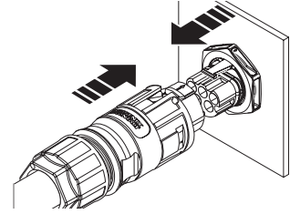
Şek. 17: AC bağlantı soketini, cihaz soketine takın
