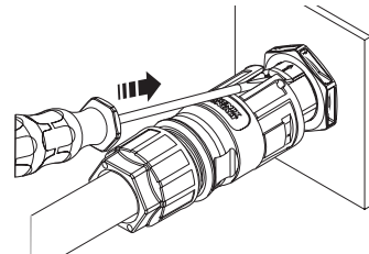
Abb. 31: AC-Anschlussstecker von dem Gerätsteckverbinder lösen
