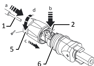
Afb. 18: Draden invoegen
