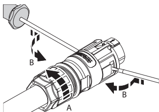
Afb. 29: Behuizing openen en kabels losmaken
