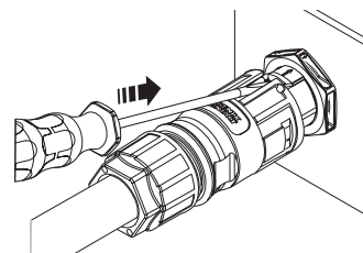
Afb. 31: AC-aansluitstekker van de stekerverbinding van het apparaat scheiden
