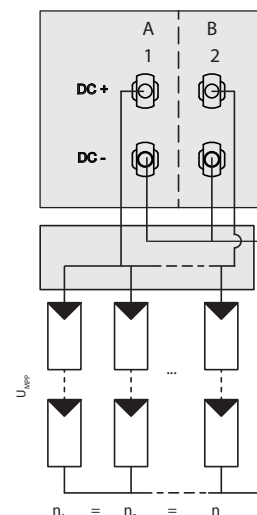
Rys. 23: Po jednym generatorze równoległym na obydwu trackerach MPP
