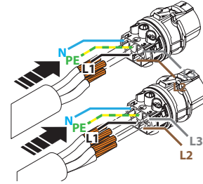
Şek. 13: Diğerinin kontaklı fişe bağlanması
