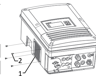
Rys. 27: Wymontowanie wentylatora
