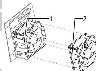
Fig. 28: Desconectar o ventilador
