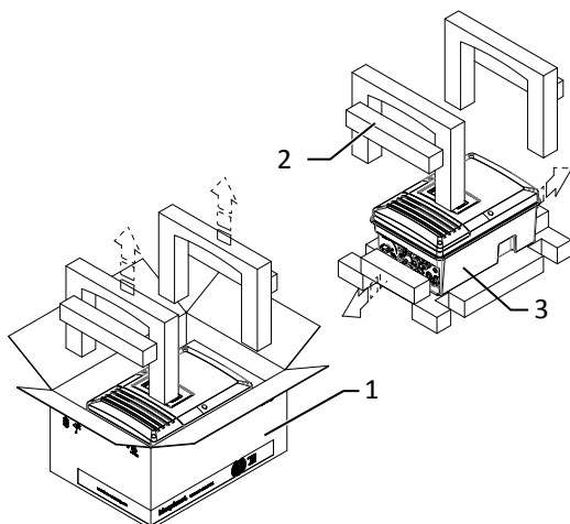
Rys. 5: Wypakowanie urządzenia
