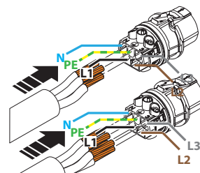
Rys. 13: Podłączanie żył do nośnika stykowego
