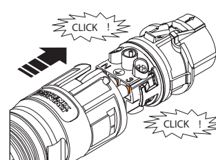
Fig. 16: Presione el portacontactos en la carcasa
