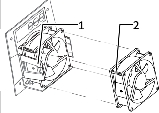
Şek. 28: Fanın çıkarılması
