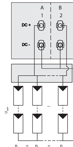
Abb. 23: Ein Generator parallel auf beiden MPP-Trackern
