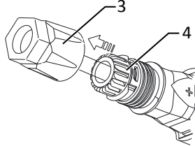
Şek. 19: Elemanın kovana geçirilmesi
