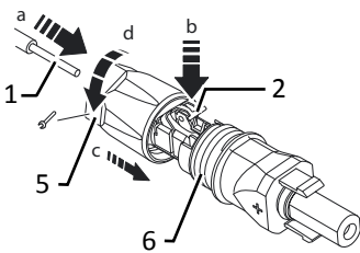
Şek. 18: Damarların içeri sokulması
