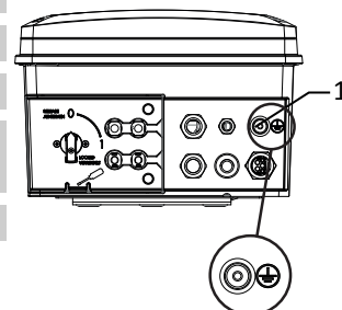
Abb. 25: Zusätzlicher Erdungspunkt
