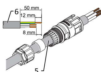
Fig. 12: Descarnar o cabo
