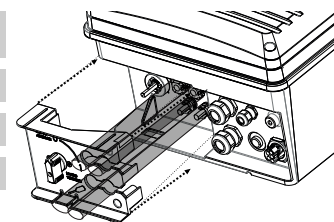
Afb. 26: Deksel van de aansluiting sluiten
