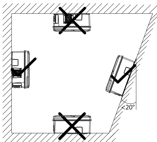
Afb. 4: Toegestane opstelstand
