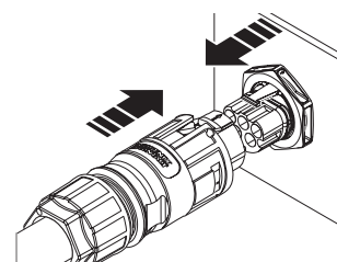
Fig. 17: Encajar el conector de CA con el conector del equipo
