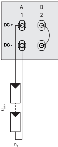
Fig. 22: Ligação em paralelo com adaptador Y, curto-circuito no tracker MPP B não usado
