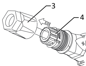
Afb. 19: Inzetstuk in huls schuiven
