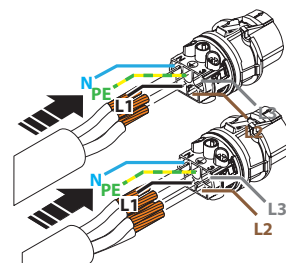
Afb. 13: Aders op contactdrager aansluiten
