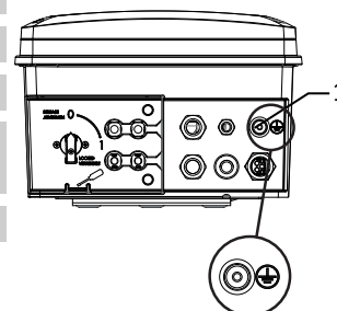
Fig. 25: Ponto de ligação à terra adicional
