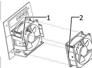
Imm. 28: Estrarre la ventola
