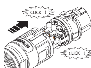
Rys. 16: Wcisnąć nośnik stykowy w obudowę
