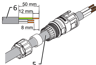
Rys. 12: Zdejmowanie izolacji z przewodów
