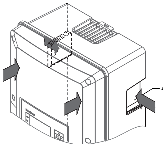
III. 6: Lever l'appareil
