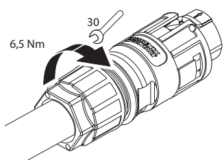
Abb. 15: Kabelverschraubung anziehen
