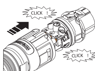
Abb. 16: Kontaktträger in Gehäuse eindrücken
