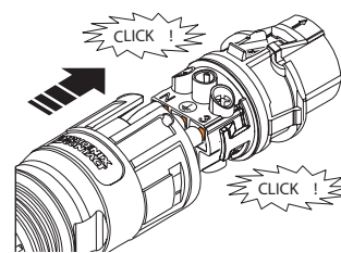
Şek. 16: Kontaklı fişin muhafazaya bastırılması
