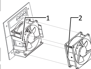
Rys. 28: Odłączanie wentylatora
