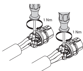
Abb. 14: Schrauben am Gehäuse anziehen
