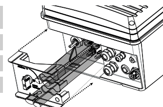
Rys. 26: Zamykanie pokrywy przyłączeniowej
