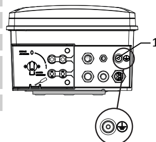
Imm. 25: Ulteriore punto di messa a terra
