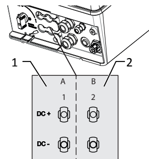
Afb. 24: Aansluiting voor DC-plus en DC-minus
