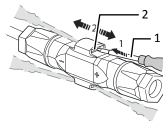
Rys. 32: Odłączanie połączenia wtykowego
