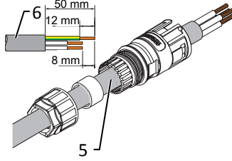
Şek. 12: Hat izolasyonunun sıyrılması
