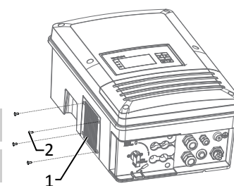
Fig. 27: Desmontaje de los ventiladores
