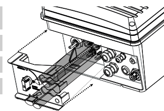
Imm. 26: Chiudere il coperchio
