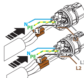
III. 13: Connecter les fils au bornier
