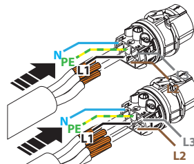
Abb. 13: Adern an Kontaktträger anschließen
