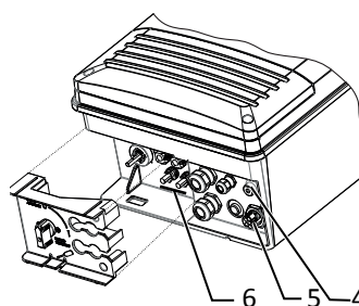
Fig. 10: Visualizar a área de conexão
