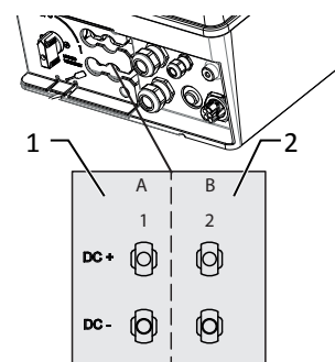
Fig. 24: Conexión para CC-positivo y CC-negativo
